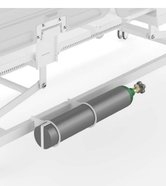
Suporte para Cilindro ACO 23
